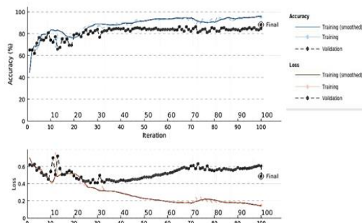
شکل ۱۱- نتایج حاصل دومین نوع معماری برای ۳۱۰ داده
