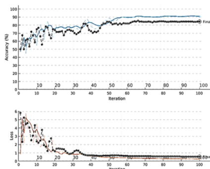
شکل ۱۲- نتایج حاصل دومین نوع معماری برای ۳۱۰ داده
