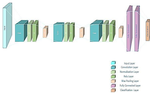
شکل ۷- سومین معماری شبکه‌های عصبی کانولوشن در حالت دو کلاسه
