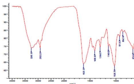
شکل ۹- طیفسنجی FT-IR از توده زیستی قارچ لنتینوس/ادودس
