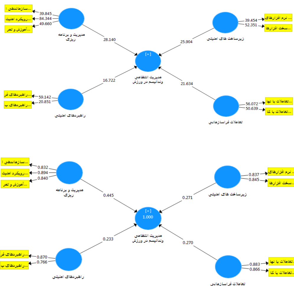
شکل ۱- مدل در حالت تخمین ضرایب استاندارد و مدل برآورد آماری
