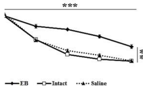
شکل ۴- نتایج آزمون ماز آبی موریس در طی ۶ روز آموزش بین گروه‌های سالین و MS را نشان می‌دهد (مقادیر نشان دهنده Means± SEM (*P≤0.05; ***P≤0.001). آزمون آماری ANOVA Repeated measure
