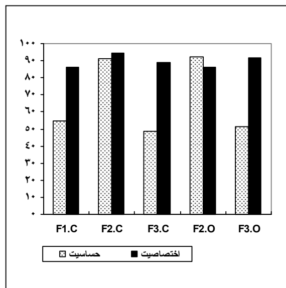
نمودار شماره ۳- ارزیابی فاسیولا هپاتیکا با روش کانتر
