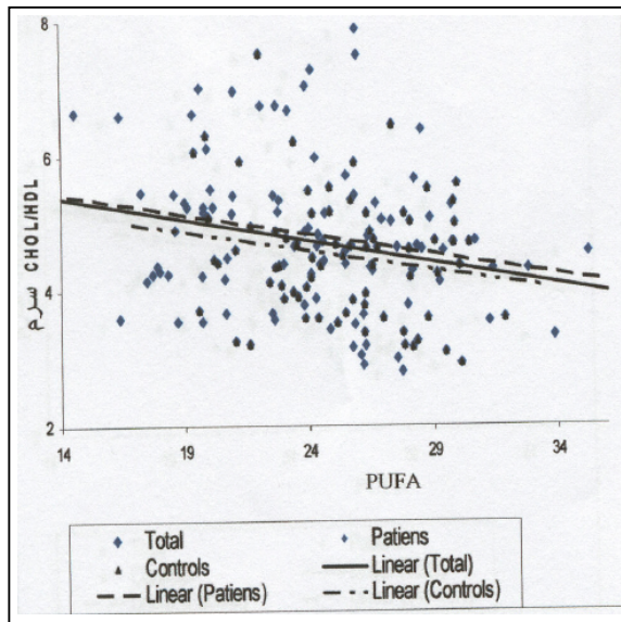
نمودار شماره ۱ - همبستگی PUFA سرم با \frac{Chol}{HDL} سرم در کل افراد مورد مطالعه ( P=0/02 ، r=-0/235 ، گروه شاهد ( P=0/10 ) و گروه بیمار ( r=-0/226 ، P=0/03 ))
