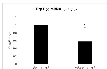
* اختلاف آماری معنی‌دار با گروه دیابت کنترل ( p \leq 0.001 ) شکل ۳- میزان نسبی mRNA ژن Drp1 در بافت بطن چپ دو گروه در پس آزمون
