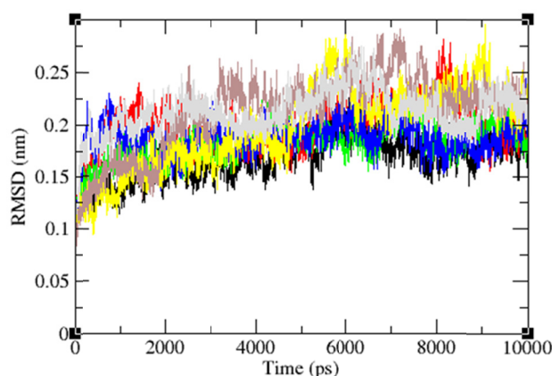
شکل ۶- نمودار تغییرات RMSD کمپلکس‌های پروتئین و پپتید در طول شبیه سازی. در این نمودارها پایین‌ترین میزان RMSD برای پپتید FLWGPRALA به رنگ مشکی و ناپایدارترین پپتید مربوط به پپتید NYKRCFPVI به رنگ زرد نشان داده شده است. پپتید VDELAHFLL (آبی)، پپتید GVDPASNTY (خاکستری)، پپتید EVDPASNTY (قرمز)، پپتید KVLHVVRV (قهوه ای) نمایش داده شده است.
