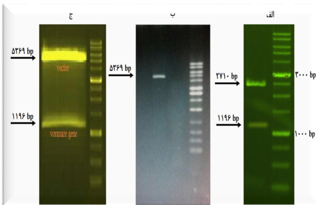
شکل ۲- مراحل کلونینگ. الف) ژل هضم دوگانه با آنزیم‌های محدودکننده NdeI و XhoI وکتور نو ترکیب pUC57 : باند مربوط به پلاسمید خطی pUC57، باند مربوط به ژن جدا شده از پلاسمید بعد از هضم آنزیمی ب) پلاسمید pET28a خطی شده بوسیله هضم آنزیم‌های محدود کننده NdeI و XhoI ج) ژل فرایند هضم دوگانه با آنزیم‌های محدودکننده NdeI و XhoI پلاسمید خطی شده در ناحیه بین 5000 bp مشخص است.
