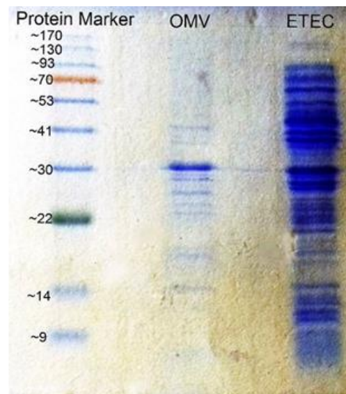
تصویر ۲- الگوی الکتروفوریتیک SDS-PAGE از روش سوم جداسازی وزیکول‌های غشاء خارجی، دامنه باندهای وزیکول‌های غشائی از ۴۱-۱۴ کیلودالتون است.
