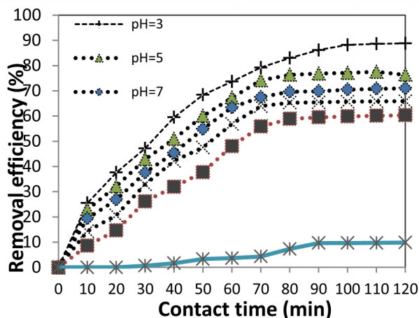
شکل ۴ ب- کارایی حذف فتوکاتالیستی پنتاکلروفنل در pH متغیر و زمان تماس ۱۲۰ دقیقه (با احتساب جذب اولیه و دوز نانو ذره=۰/۶ گرم) و کارایی اشعه UV به تنهایی در زمان تماس ۱۲۰ دقیقه (غلظت پنتاکلروفنل=۳۰ میلیگرم بر لیتر)
