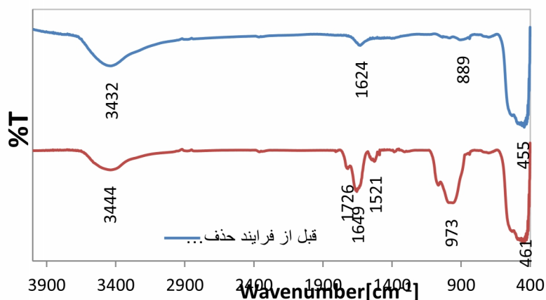
شکل ۳- آزمون FTIR نانو ذرات اکسید روی مورد استفاده قبل (الف) و بعد (ب) از فرایند حذف پنتاکلروفنل
