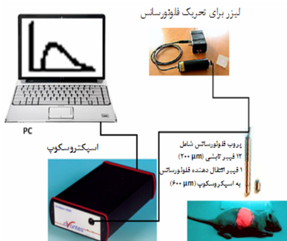
شکل شماره ۱- سیستم طراحی شده برای اندازه‌گیری سیگنال فلئورسانس به طور غیرتهاجمی و از روی سطح بافت.
