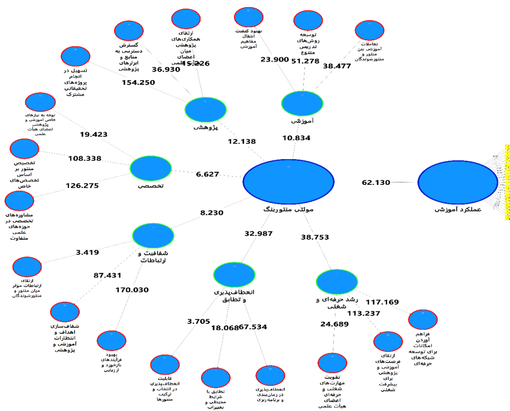
نمودار ۲- تاثیر مولتی، متتورینگ بر عملکرد آموزش، در حالت معنی، داری ضرایب مسیر
