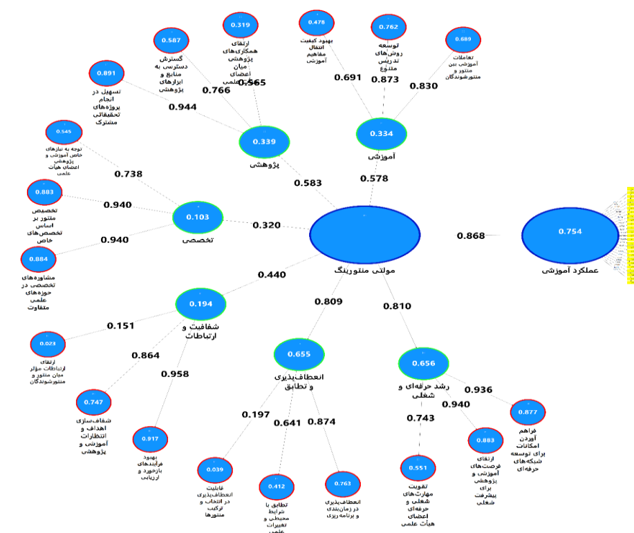
نمودار ۱- تأثیر مولتی منتورینگ بر عملکرد آموزشی در حالت تخمین ضرایب مسیر
