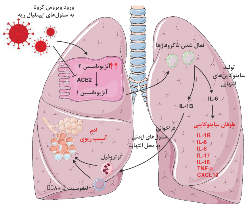
شکل ۳- ورود ویروس کرونا به ریه و ایجاد التهاب. ویروس کرونا با ورود به سلول‌های اپیتلیالی ریه و کاهش فعالیت آنزیم مبدل آنژیوتانسین باعث افزایش سطح آنژیوتانسینوژن ۲ می‌شود. در ادامه فرایندهای التهابی آغاز و ماکروفاژها شروع به تولید اینترلوکین-۱بتا و اینترلوکین-۶ کرده و با تحریک تولید هرچه بیشتر اینترلوکین‌ها و فاکتور نکروز تومور، طوفان سایتوکاینی اتفاق می‌افتد. همزمان، فراخوانی نوتروفیل‌ها و لنفوسیت‌ها با تشدید التهاب باعث ادم و آسیب ریوی می‌شود. (تصویر اصالت دارد)
