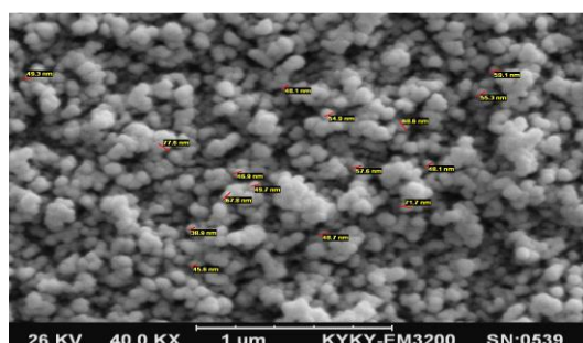
شکل ۵ - تصویر SEM نانوکامپوزیت های سلولز-گرافن
