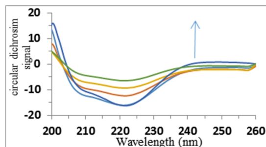
نمودار ۶- نمودار CD رسم شده برای پروتئین آلبومین با غلظت ۲ میکرومولار در حضور غلظت‌های مختلف نانوذرات الماس (صفر، ۱۵، ۲۰، ۱۰۱، ۲۰۰ میکروگرم در میلی‌لیتر).
