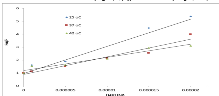
نمودار ۵- نمودار اشترن والمر در نتیجه تعامل نانوذرات الماس با پروتئین آلبومین در دماهای مختلف ۲۹۸، ۳۱۰، ۳۱۵ درجه کلون
