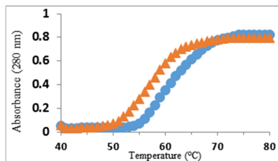
نمودار ۷- نقطه ذوب پروتئین آلبومین در حضور و عدم حضور نانوذرات الماس در pH = ۷/۵، ۱۰ میکرومولار بافر فسفات در ۳۹۸ نانومتر.
