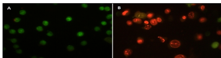
نمودار ۳- نتایج رنگ‌آمیزی آکریدین اورنج/اتیدیوم بروماید: A گروه سالم، B گروه سلول سرطان سینه (MCF-7) تیمار شده با نانوذرات الماس
