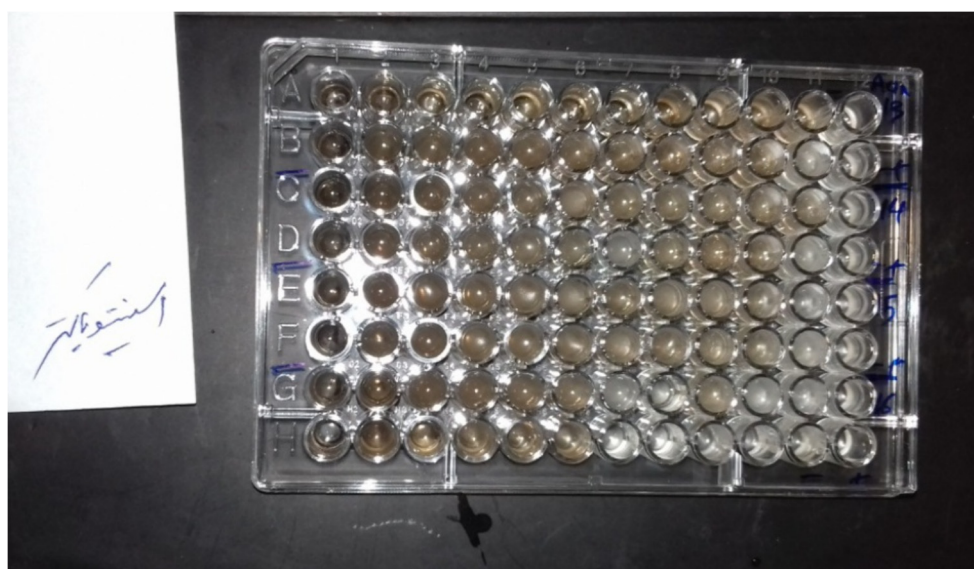
تصویر ۱- چاهک‌های میکروداپلو شن آنتی‌بیوتیکی به ترتیب: ردیف اول: تیکارسیلین، ردیف دوم: جنتامایسین، ردیف سوم: سیپروفلوکساین، ردیف چهارم: سفپیم، ردیف پنجم: پیپراسیلین، ردیف ششم: آمیکاسین، ردیف هفتم: توبرامایسین، ردیف هشتم: کولیستین.
