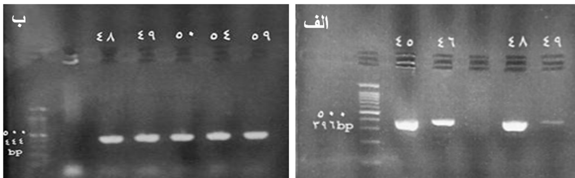
شکل ۳- باند ۳۹۶ جفت بازی مربوط به ژن Exo A نمونه‌ی ۴۵ و ۴۶ ادرار، نمونه ۴۸ و ۴۹ زخم (الف) و باند ۴۴۴ جفت بازی مربوط به ژن Exo S نمونه ۴۸ و ۴۹ - زخم، نمونه ۵۰ و ۵۹ - ادرار و نمونه ۵۴ - خون (ب).
