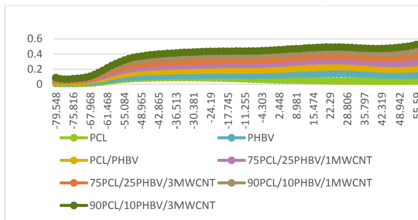
شکل ۸- منحنی اتلاف \delta \text{ Tan} از PCL، PHBV، PCL/PHBV، 75PCL/25PHBV/1,3MWCNT، 90PCL/10PHBV/1,3MWCNT
