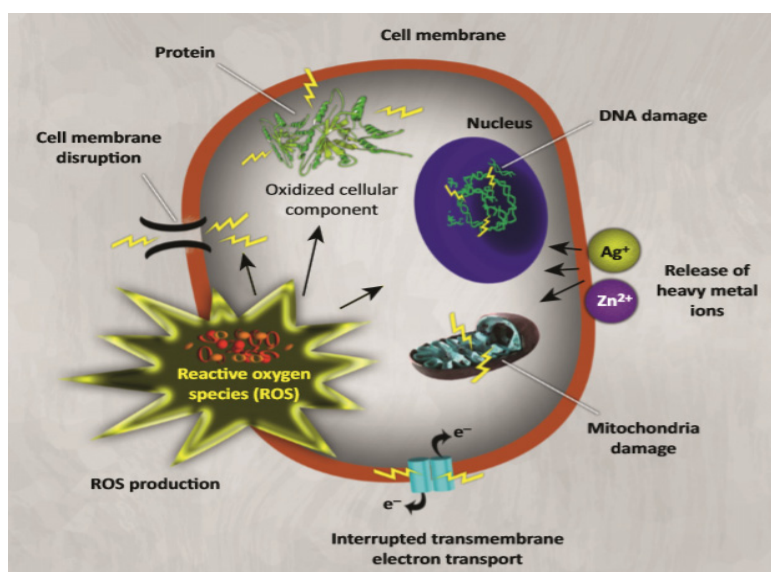
شکل ۴- مکانیسم های سمیت نانوذرات (NPs) علیه باکتری ها (۴۹)
