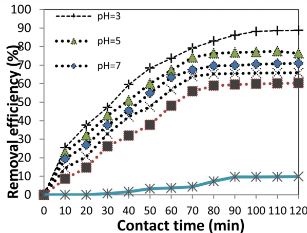
شکل ۴ ب- کارایی حذف فتوکاتالیستی پنتاکلوروفنل در pH متغیر و زمان تماس ۱۲۰ دقیقه (با احتساب جذب اولیه و دوز نانو ذره=۰/۶ گرم) و کارایی اشعه UV به تنهایی در زمان تماس ۱۲۰ دقیقه (غلظت پنتاکلوروفنل=۳۰ میلیگرم بر لیتر)
