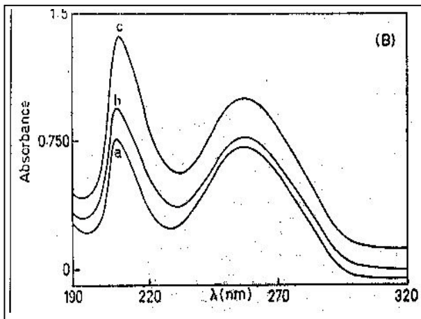
(B) - طیف جذبی DNA رشته‌ای، a- طیف جذبی DNA در برابر بافر تریس، b- طیف جذبی کمپلکس DNA-LMG در برابر غلظتهای به ترتیب ۰/۵ و ۲ میلی مولار LMG
