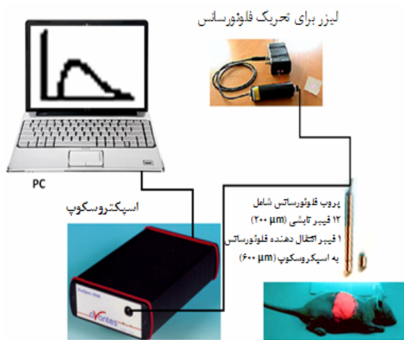
شکل شماره ۱- سیستم طراحی شده برای اندازه‌گیری سیگنال فلئورسانس به طور غیرتهاجمی و از روی سطح بافت.
