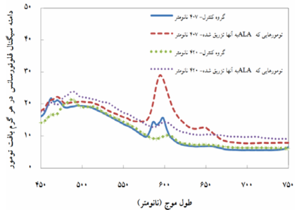
شکل شماره ۲- مقایسه دو طول موج ۴۰۷ nm و ۴۲۰ nm برای تحریک فلئورسانس PpIX.
