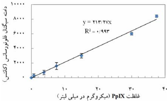
شکل شماره ۷- منحنی استاندارد PpIX تعیین شده به روش فلئورسانس اسپکتروسکوپی. (داده‌ها نماینگر میانگین سه بار اندازه‌گیری \pm خطای استاندارد است) نتایج در طول موج نشری ۶۳۵ nm و طول موج تحریک ۴۰۵ nm اخذ شده است.
