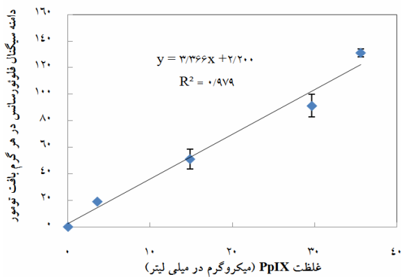
شکل شماره ۴- منحنی استاندارد PpIX. (داده‌ها نمایانگر میانگین سه بار اندازه‌گیری \pm خطای استاندارد است) سیگنال نشری به روش فلئوریمتری و در طول موج نشری ۶۰۰ nm و طول موج تحریک ۴۰۷ nm تعیین شده است.
