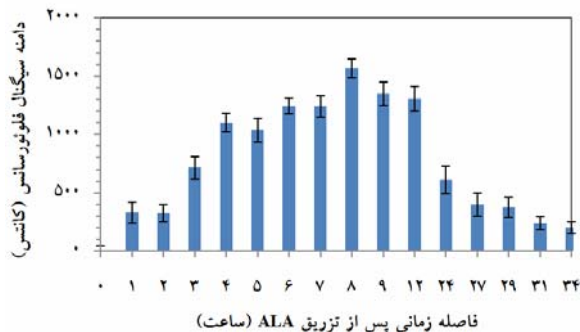
شکل شماره ۸- هیستوگرام شدت سیگنال فلئورسانس از سطح بافت تومور بر حسب فاصله زمانی پس از تزریق ALA به میزان ۲۰۰ mg/kg. داده‌ها نماینگر میانگین سه بار اندازه‌گیری از هر یک از ۳ موش \pm خطای استاندارد است. میانگین فلئورسانس ذاتی بافت قبل از تزریق ALA از تمام داده‌ها کم شده است.
