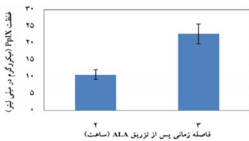
شکل شماره ۵- نمودار غلظت PpIX درون بافت تومور پس از تزریق ALA به میزان ۵۰۰ mg/kg و در زمان‌های ۲ ساعت و ۳ ساعت پس از تزریق (داده‌ها نمایانگر سه بار اندازه‌گیری \pm خطای استاندارد است).
