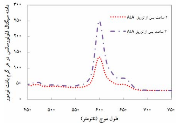
شکل شماره ۳- بررسی تأثیر فاصله زمانی بین تزریق ALA و اخذ طیف فلئورسانس بر تجمع PpIX درون تومور
