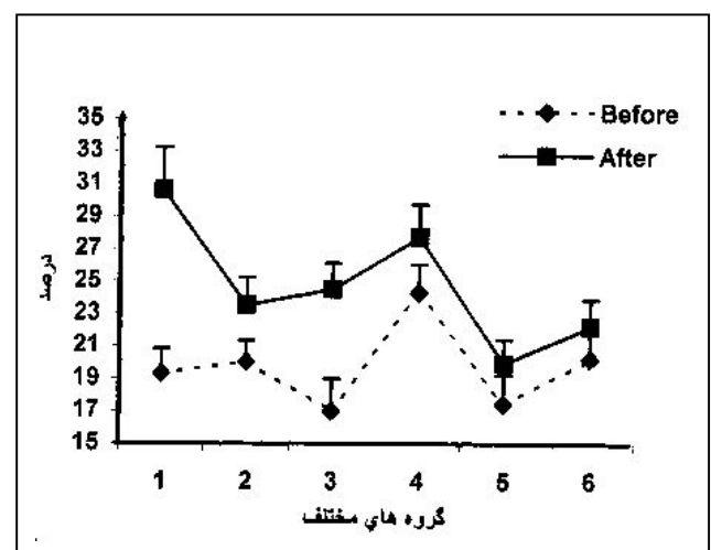
نمودار شماره ۲- تغییرات درصد اشباع ترانسفرین به صورت میانگین \pm خطای استاندارد از میانگین در مراحل قبل و بعد از درمان نشان داده شده است ( P < 0.05 ).
