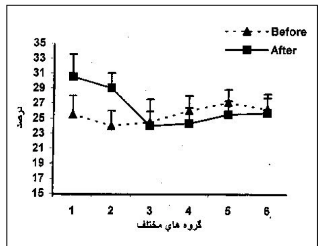
نمودار شماره ۱- تغییرات سطح هماتوکریت به صورت میانگین \pm خطای استاندارد از میانگین در مراحل قبل و بعد از درمان نشان داده شده است ( P < 0.05 ).
