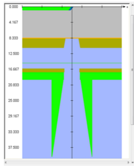
شکل ۱- سر شبیه سازی شده دستگاه درمانی ارتولتاژ نوع Stubilipan با کد BEAMnrc.
