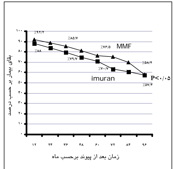
نمودار شماره ۳- بقای پیوند کلیه در ۹ سال اخیر (مقایسه بیماران تحت درمان با داروی MMF نسبت به ایموران)
