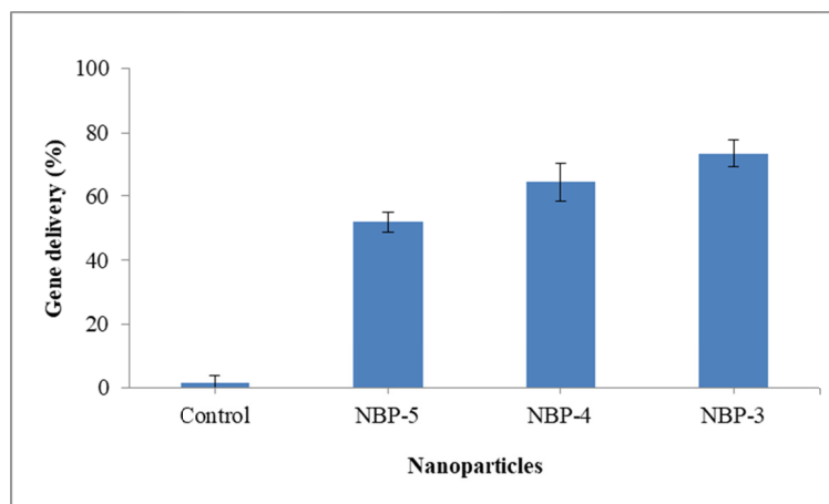
شکل ۱۰- مقایسه میانگین نتایج حاصل از دستگاه فلوسایتمتری از شمارش سلول‌های تیمار شده با نانو ذرات NBP-3، NBP-4 و NBP-5 حاوی PEI/siRNA-FAM
