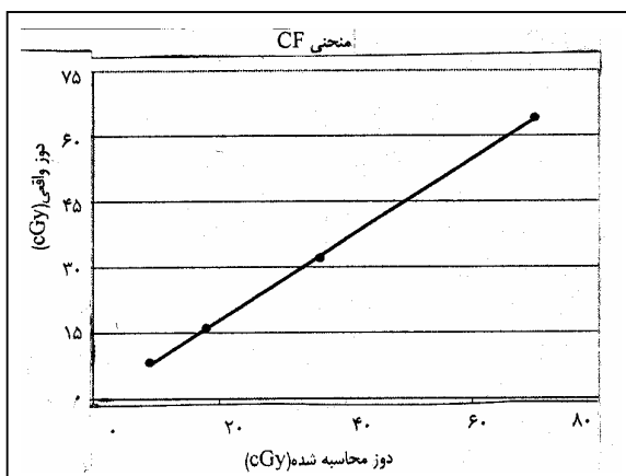
نمودار شماره ۲- منحنی ضریب تصحیح دوز واقعی به دوز محاسبه شده
