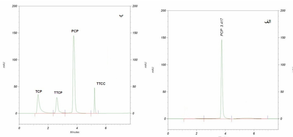
شکل ۷ الف- کروماتوگراف مربوط پنتاکلروفنل بدون تابش UV. ب- کروماتوگراف مربوط به پنتاکلروفنل و ترکیبات واسط تولیدی بعد از فرایند (trichlorophenol)TCP, (tetrachlorocatechol)TTCC, (tetrachlorophenol)TTCP.UV/ZnO
