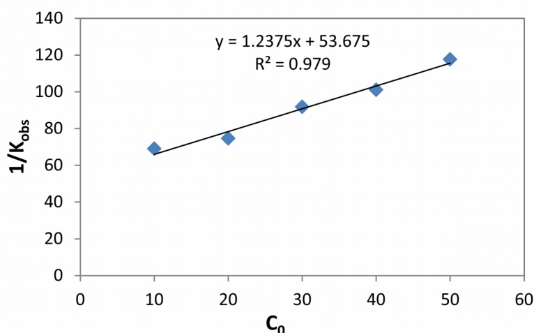
شکل ۸- سینتیک واکنش Langmuir- Hinshelwood در غلظت های مختلف پنتاکلروفنل
